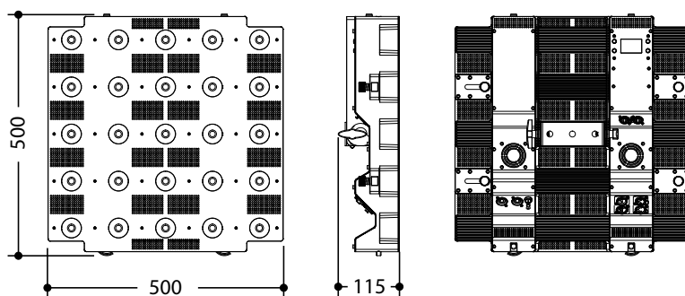
Disegno tecnico
