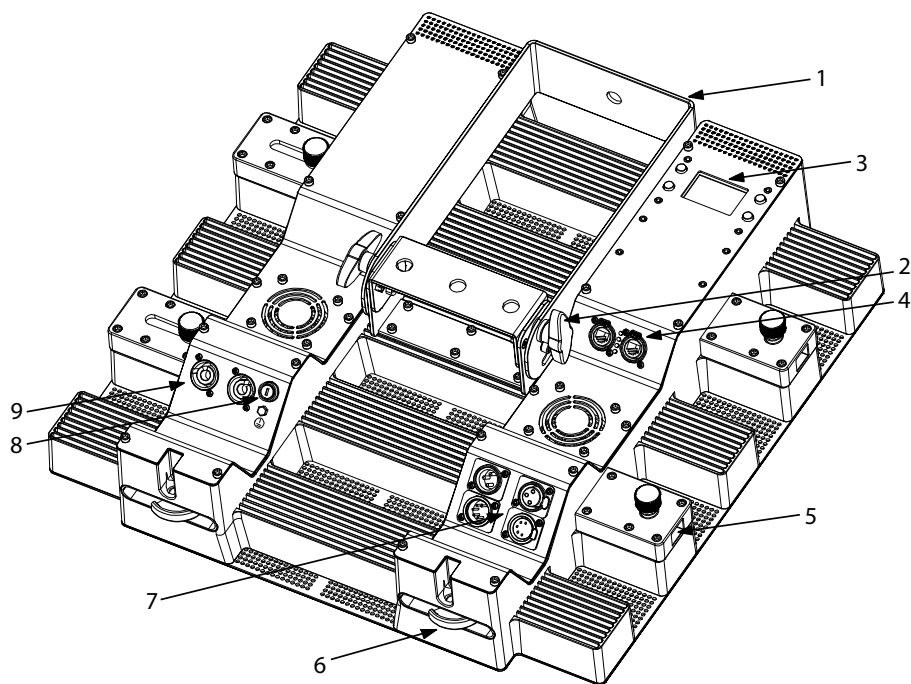
Pannello Posteriore
