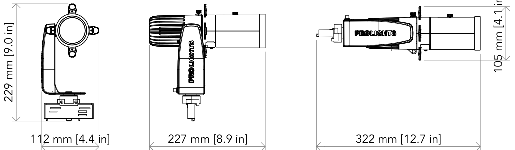
Fig.2 - Disegno tecnico
