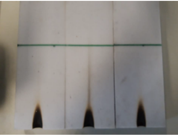
Aspecto de la muestra tras del ensayo de inflamabilidad según EN ISO 11925-2 (aplicado en borde)
